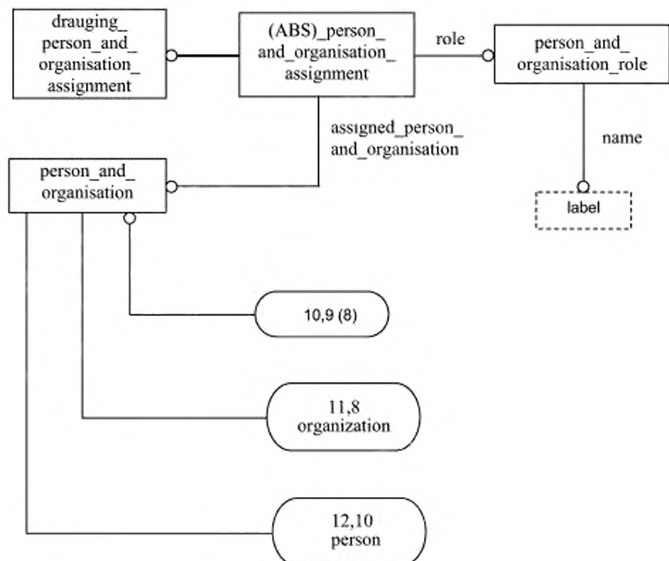
Рисунок С.10 — Расширенный листинг ПИК — EXPRESS-G диаграмма 10 из 14
