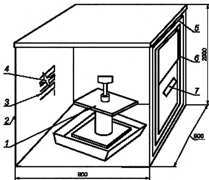
1 — станок для испытаний тары на штабелирование; 2 — теплоизолирующая камера; 3 — нагреватель; 4 — вентилятор; 5 — дверь; 6 — смотровое окно; 7 — ручка
