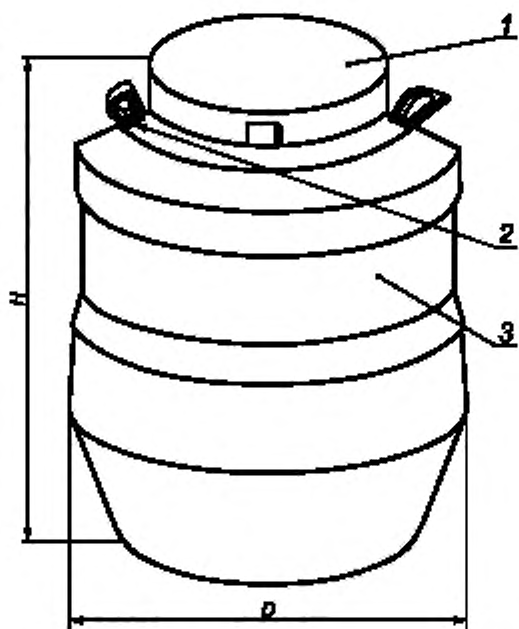
1 — крышка; 2 — ручка, прикрепленная к корпусу; 3 — корпус
