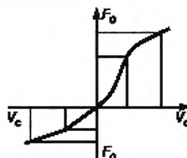
Рисунок 4 — Зависимость сопротивления амортизатора от скорости перемещения поршня
