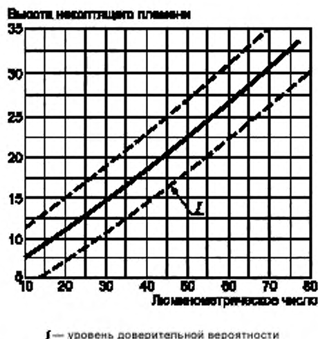
Рисунок X1.1 — Зависимость между высотой некоптящего пламени и люминометрическим числом
