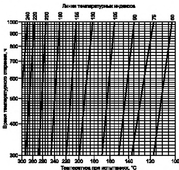
Рисунок 2J — Временное тепловое старение
