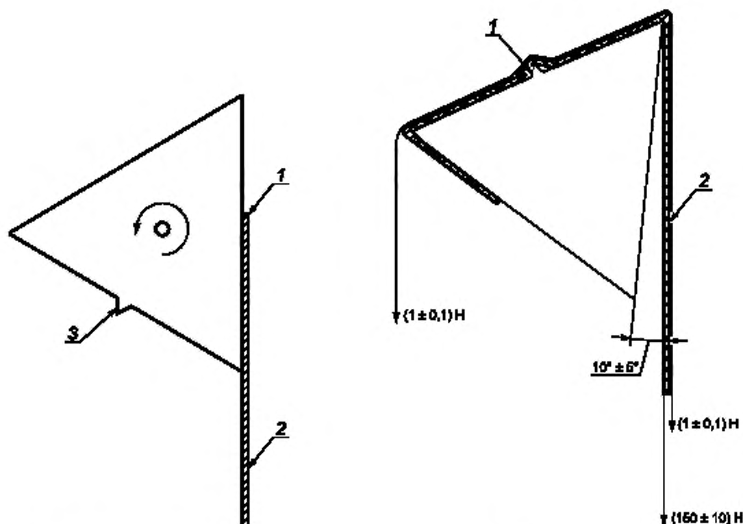
Рисунок AA.2 — Начальное положение оправки
