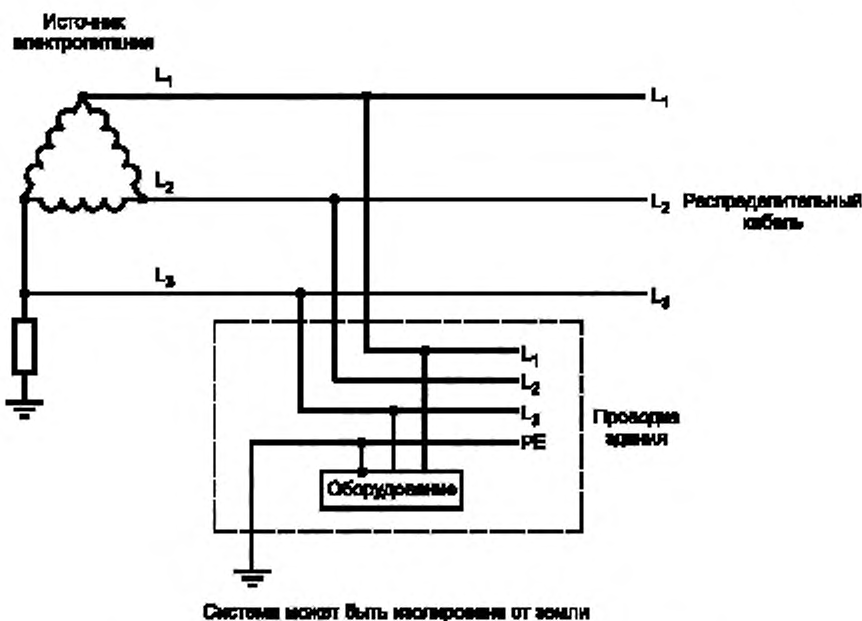
Рисунок V.8 — Пример IT-системы электропитания с тремя фазами
