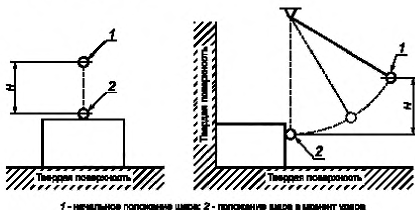
Рисунок 4А — Испытание на удар стальным шаром
