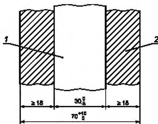
Рисунок AA.3 — Конечное положение оправки
