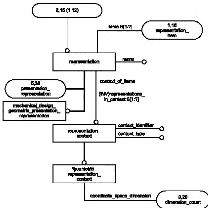
Рисунок С.2 — ПИК aic_mechanical_design_geometric_representation в формате EXPRESS-G (диаграмма 2 из 14)
