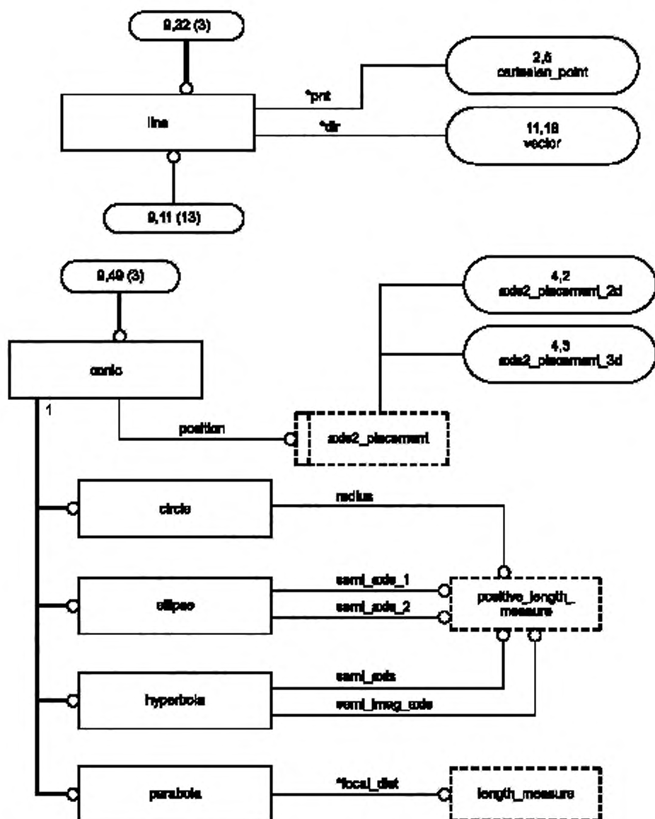
Рисунок С.9 — ПИК geometrically_bounded_surface в формате EXPRESS-G (диаграмма 9 из 18)
