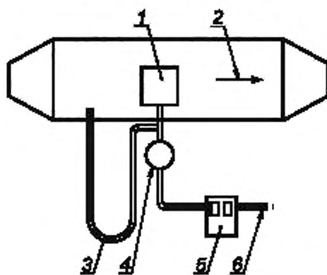
1 — испытуемый фильтр; 2 — направление потока воздуха; 3 — манометр; 4 — насос; 5 — счетчик или расходомер; 6 — сброс
