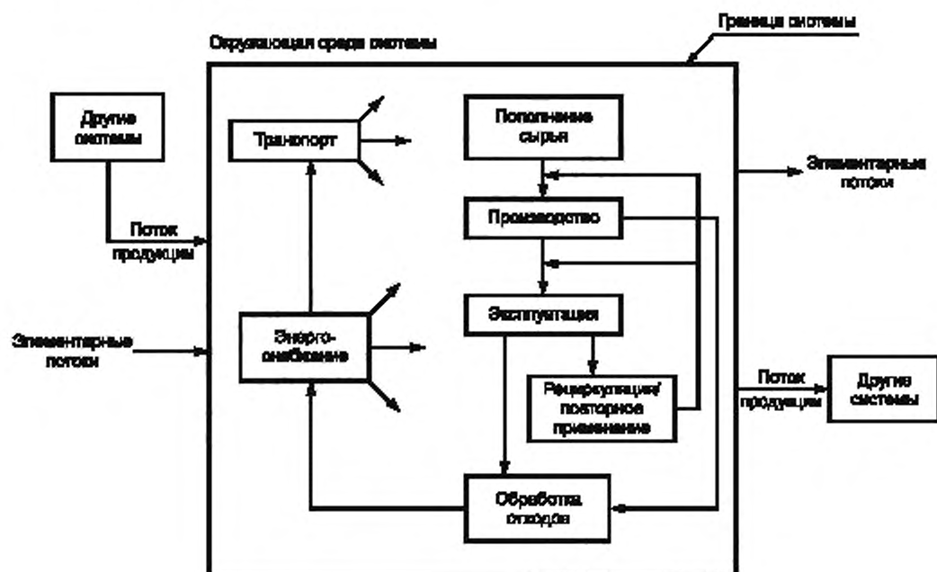
Рисунок 2 — Пример производственной системы для ОЖЦ
