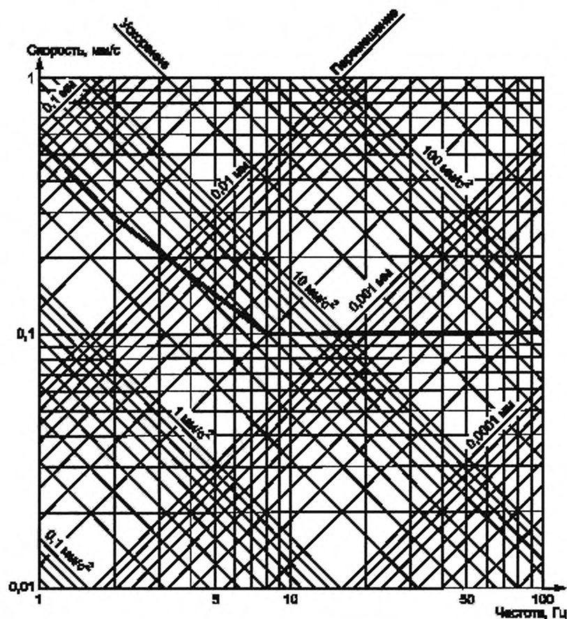
Рисунок В.1 — Кривая равной чувствительности
