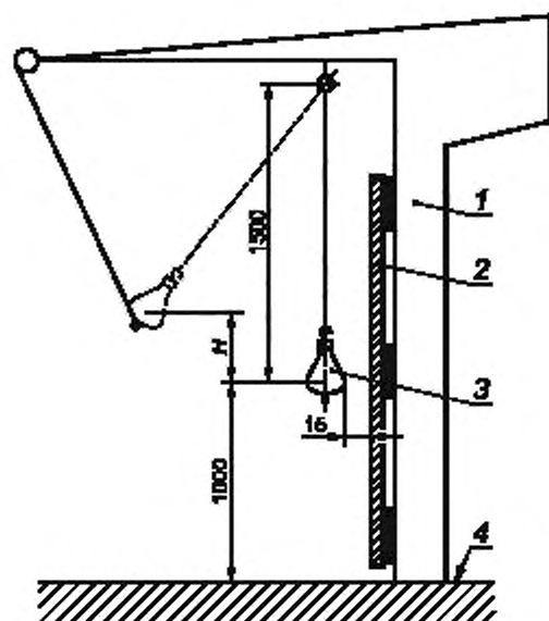
1 — рама, 2 — испытываемая стеклянная панель; 3 — маятник; 4 — уровень пола, относящийся к испытываемой стеклянной панели; H — высота падения
