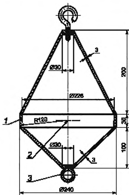
1 — ударное кольцо; 2 — базисная точка для измерения высоты падения; 3 — крепление пускового приспособления
