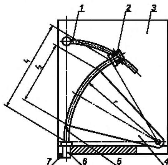
1 — направляющая; 2 — фиксатор; 3 — щит; 4 — шаблон для задания радиуса изгиба; 5 — труба; 6 — фитинг; 7 — соединительный nipple; l_1 — полная длина трубы; l_2 — длина опоры изгиба; r — радиус изгиба
