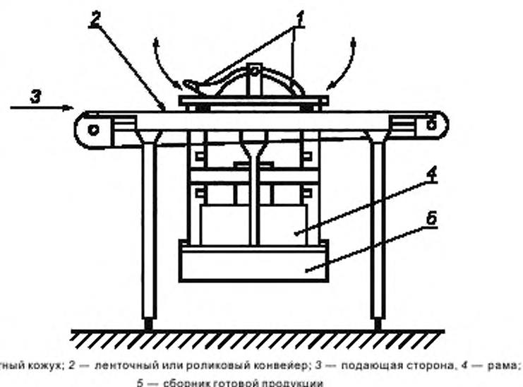
Рисунок 2 — Пила, установленная в линию
