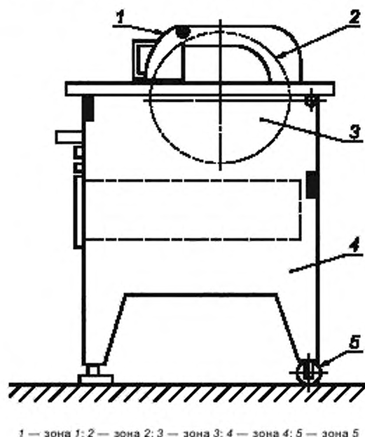
Рисунок 3 — Пила напольного типа — опасные зоны
