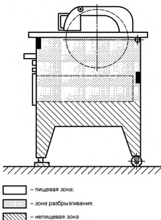
Рисунок 10 — Гигиенические области в пилах
