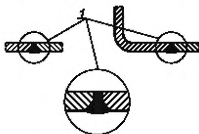
Рисунок А.1 — Пищевая зона
