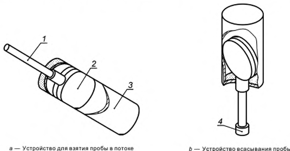
1 — кварцевая трубка; 2 — разъемная форма; 3 — картон; 4 — колпачок
