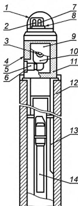
1 — защитные колпачки; 2 — кислородная ячейка; 3 — термopapa остановки ликвидуса; 4 — картонная трубка; 5 — раскислитель; 6 — боковое накопление; 7 — термopapa; 8 — железный контактный электрод; 9 — металлическая пластина охлаждения; 10 — камера для образца; 11 — песчаное тело; 12 — картонная труба; 13 — выпуск газа; 14 — соединение
