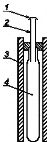
б — Вакуумный пробоотборник
