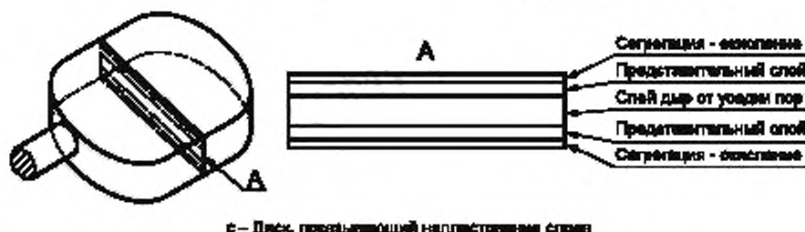
Рисунок А.2 — Примеры образцов в виде диска со штырьком
