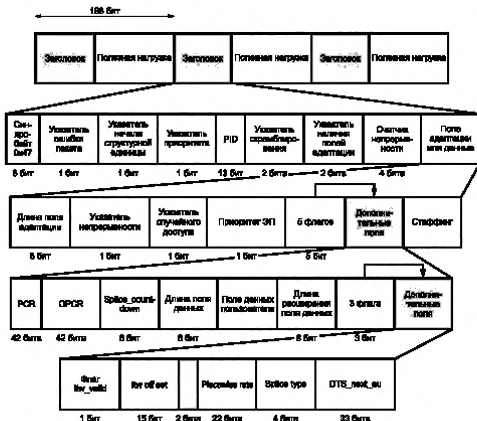
Рисунок А.2 — Структура основных полей транспортного потока MPEG
