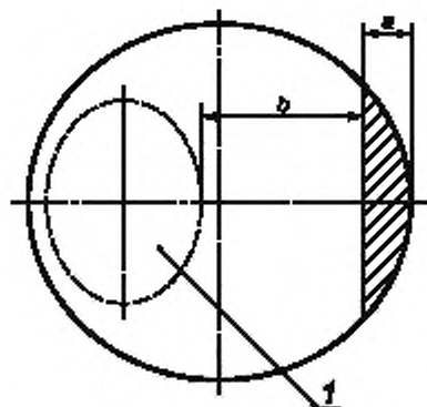
1 — пространство, перекрываемое месильным органом; а — расстояние между внутренним ободом дежи и внутренней частью защитного устройства; b — расстояние по горизонтали между внешней частью защитного устройства и ближайшей точкой опасной зоны, т. е. пространство, перекрываемое движением месильного органа
