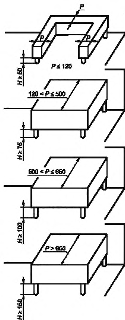
Рисунок А.18 — Станины для машин
