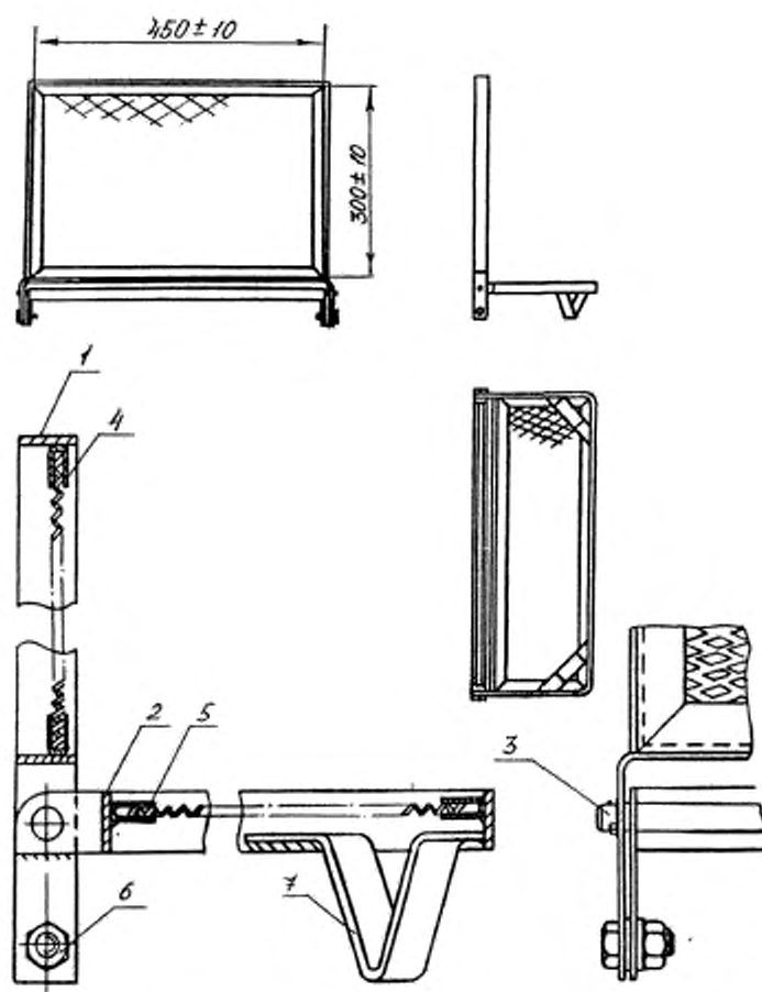
1, 2 — стальные рамы; 3 — шарнир; 4, 5 — стальные сетки; 6 — болт; 7 — ножка
