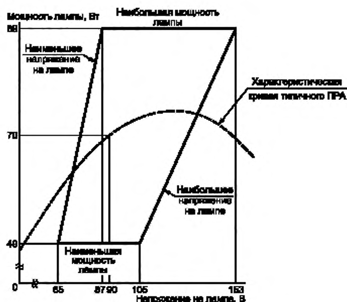
Рисунок 5.6 — Предельные рабочие характеристики ламп номинальной мощностью 70 Вт с прозрачной трубчатой, эллипсоидной прозрачной или с диффузным покрытием колбой
