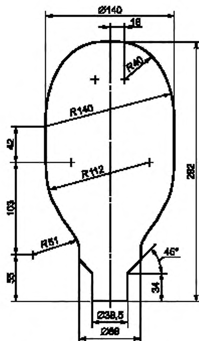
Рисунок G.4 — Эллипсоидная лампа мощностью 400 Вт
