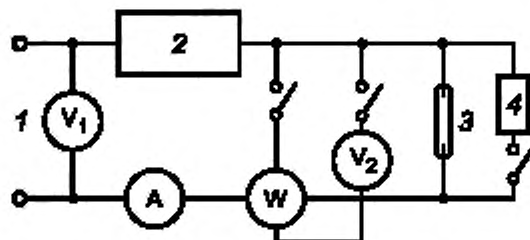
1 — источник питания; 2 — ДОО; 3 — лампа; 4 — ЗУ (тип 1)
