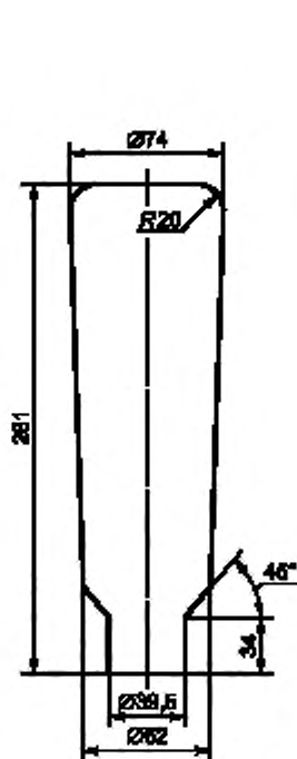
Рисунок G.1 — Трубчатая лампа мощностью 250 Вт
