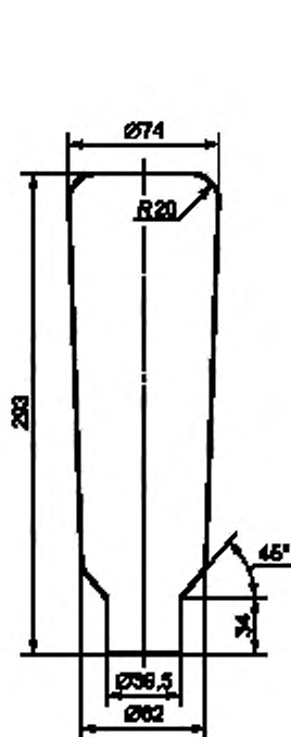
Рисунок G.3 — Трубчатая лампа мощностью 400 Вт
