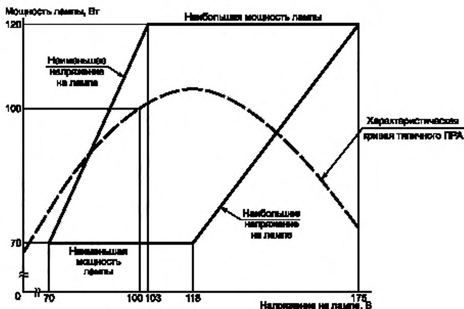
Рисунок 5.5 — Предельные рабочие характеристики ламп номинальной мощностью 100 Вт с трубчатой прозрачной или эллипсоидной с диффузным покрытием колбой
