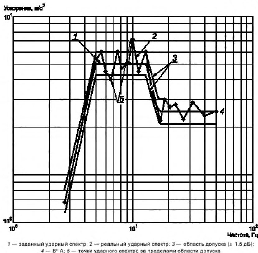
Рисунок 3 — Типичный график ударного спектра (в логарифмическом масштабе)
