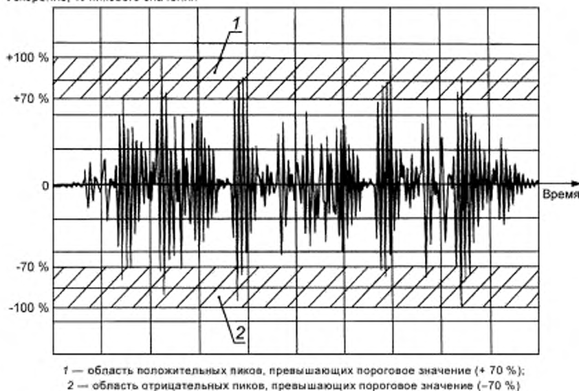
Рисунок 1 — Пример отклика осциллятора на заданный временной сигнал возбуждения
