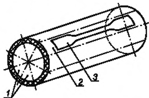
1 — сектор; 2 — полоса; 3 — испытуемый образец
