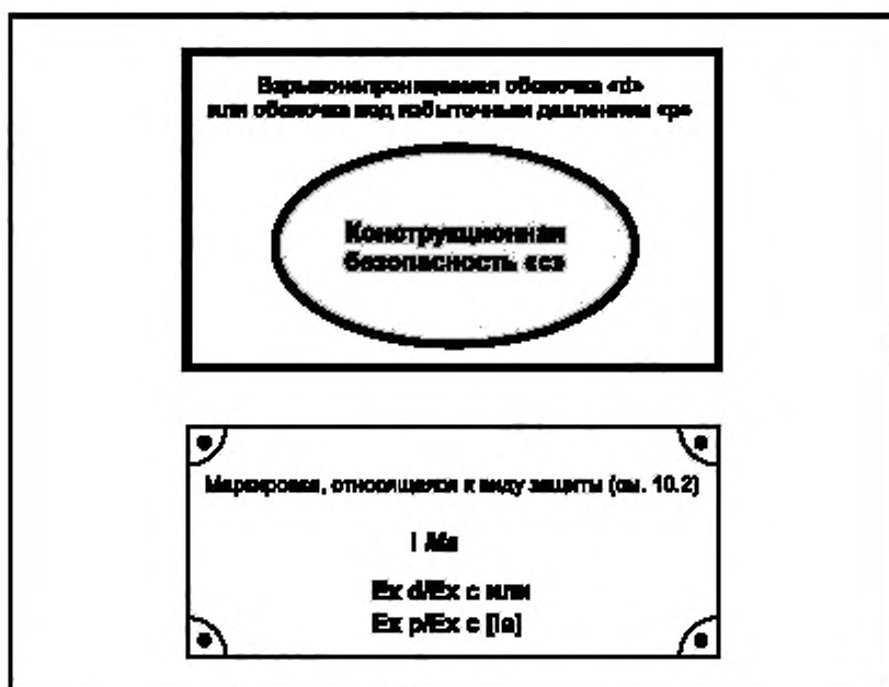
Рисунок 5 — Оборудование уровня взрывозащиты Ma (конструкционная безопасность «c» внутри взрывонепроницаемой оболочки «d» или оболочки под избыточным давлением «p»)
