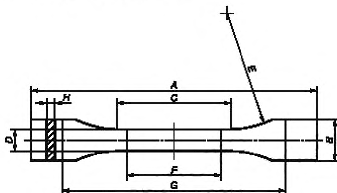
Рисунок 1 — Испытуемый образец типа 1
