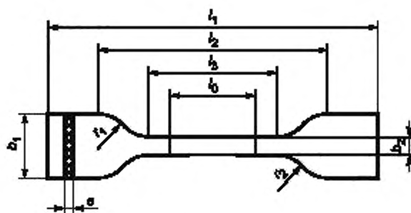
Рисунок 1 — Образец типа 1
