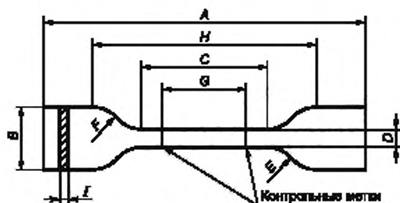
Рисунок 2 — Испытуемый образец типа 2
