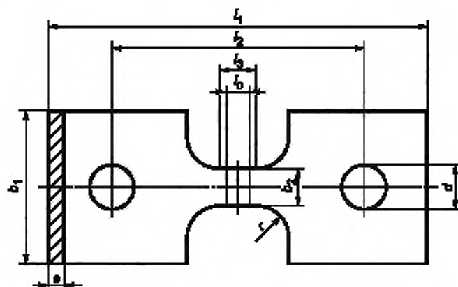
Рисунок 3 — Образец типа 3
