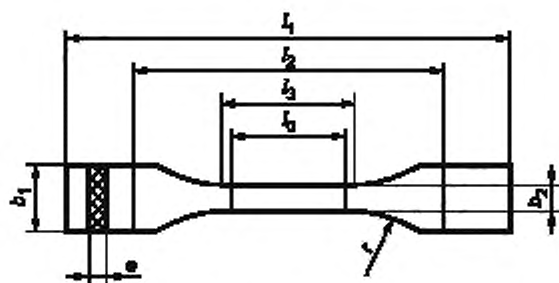
Рисунок 2 — Образец типа 2
