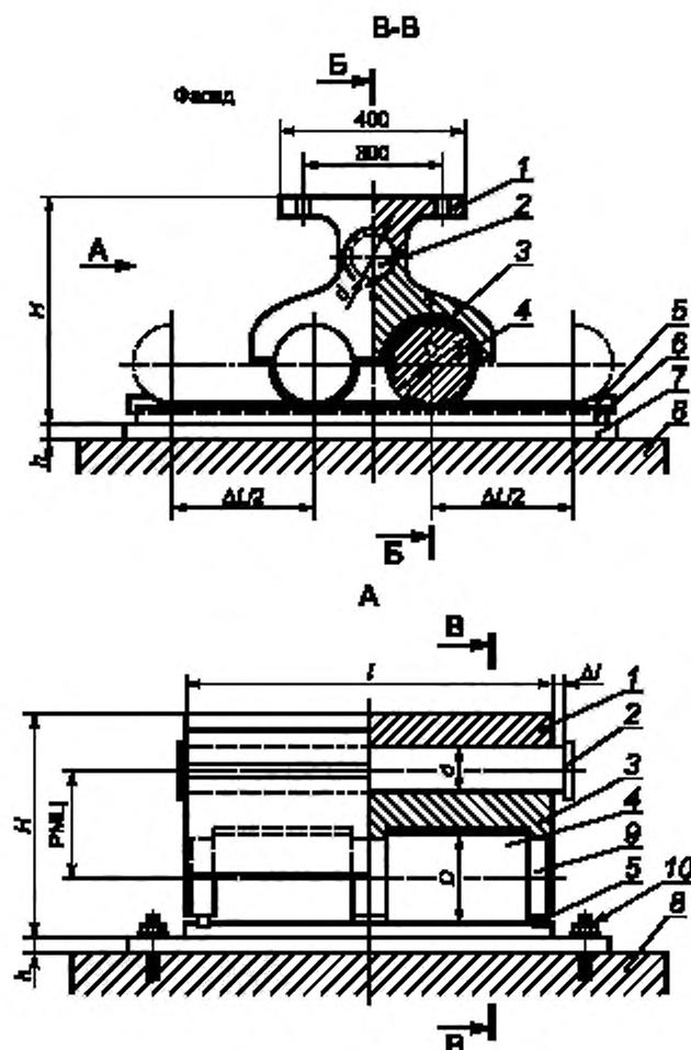
H — высота опорной части; РМЦ — расстояние между осями шарнира и катков; h — толщина подопорного листа; D — диаметр катков; d — диаметр оси-шарнира; l — длина балансира, катков, опорного листа; l + \Delta l — длина оси-шарнира; \Delta l и \Delta L — поперечное и продольное перемещение пролетного строения; 1 — верхний балansir; 2 — ось-шарнир; 3 — нижний балansir; 4 — каток; 5 — противоугол; 6 — опорный лист; 7 — лист — закладная деталь; 8 — подферменная площадка; 9 — цапфа; 10 — анкерный болт
