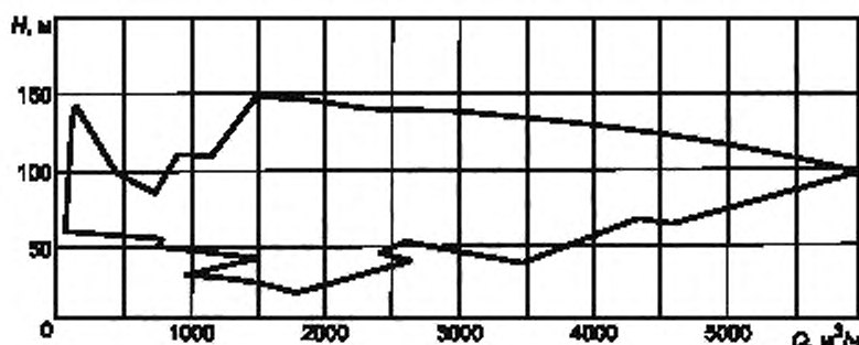
Рисунок В.2 — Совмещенные поля Q - H горизонтальных подлорных насосов
