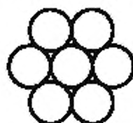
Рисунок 1 — Конструкция каната 1 × 7(1 + 6)
