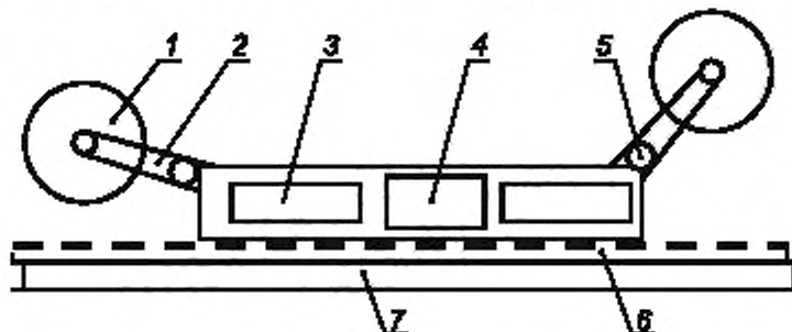
1 — шнек срезцами; 2 — поворотный редуктор; 3 — отделение редуктора; 4 — взрывозащищенное распределительное устройство; 5 — взрывозащищенный шнековый электродвигатель; 6 — расположение ременной передачи; 7 — забойный скребковый конвейер
