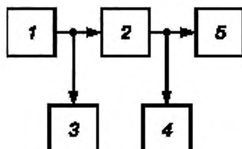
1 — низкочастотный генератор сигналов; 2 — измеряемое звено; 3, 4 — вольтметры, 5 — номинальное сопротивление нагрузки — резистор
