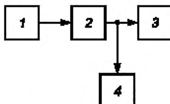
1 — резистор — эквивалент сопротивления источника; 2 — измеряемый тракт или звено, 3 — номинальное сопротивление нагрузки — резистор; 4 — псифометр
