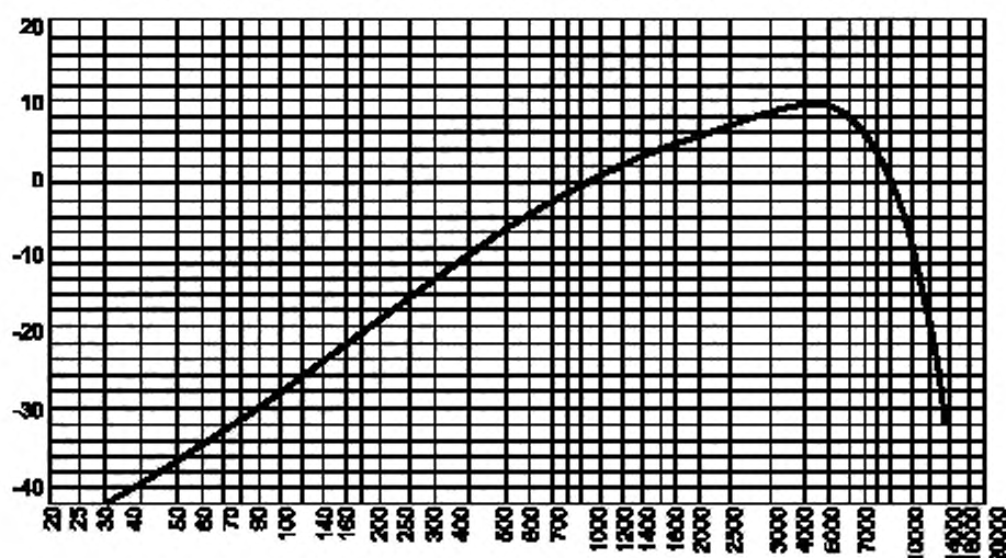
Рисунок 2 — График АЧХ псофометрического фильтра в соответствии с [5]
