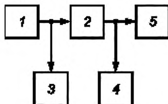
1 — низкочастотный генератор сигналов; 2 — измеряемое звено; 3 — вольтметр; 4 — измеритель нелинейных искажений или анализатор спектра; 5 — номинальное сопротивление нагрузки — резистор
