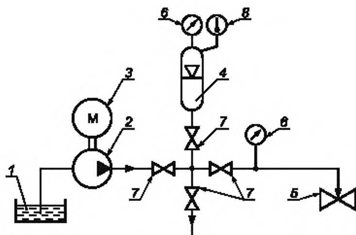
1 — емкость для забора воды; 2 — насос (допускается применять другие технические средства); 3 — электродвигатель; 4 — гидропневмоаккумулятор; 5 — испытуемая арматура; 6 — прибор для измерения давления; 7 — запорно-регулирующий клапан; 8 — термометр
