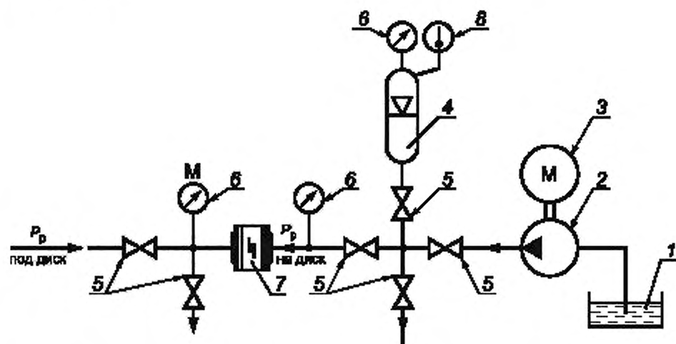
Рисунок В.6 — Принципиальная схема стенда для испытаний обратной арматуры на герметичность затвора и проверку функционирования
