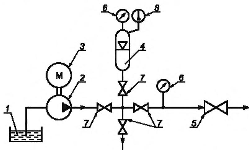
1 — емкость для забора воды; 2 — насос (допускается применять другие технические средства); 3 — электродвигатель; 4 — гидропневмоаккумулятор; 5 — испытуемая арматура; 6 — прибор для измерения давления; 7 — запорно-регулирующий клапан; 8 — термометр
