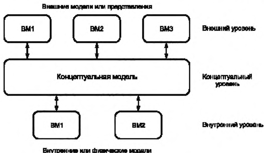
Рисунок 3 — Трёхсхемная архитектура
