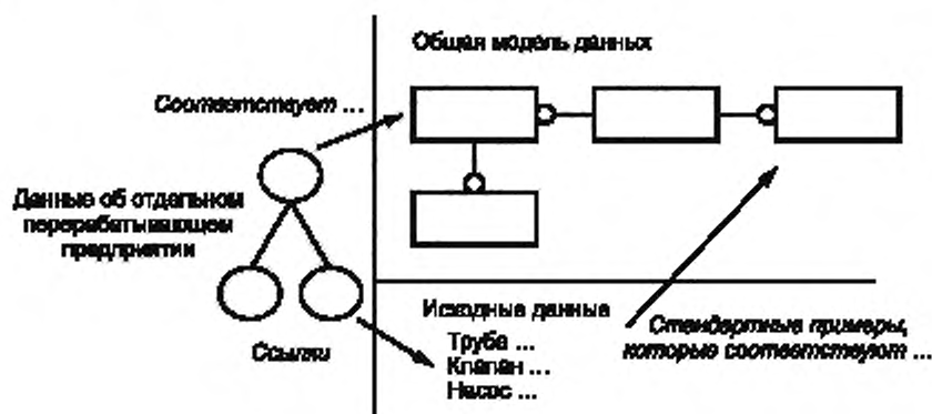
Рисунок 2 — Архитектура
