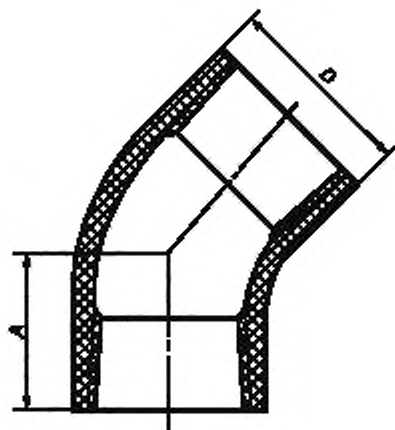
Рисунок 5 — Отвод с углом поворота 45°
