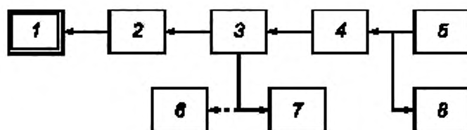
1 — испытываемое оборудование; 2 — аттенюатор; 3 — делитель мощности; 4 — высокочастотный генератор сигналов; 5 — низкочастотный генератор сигналов; 6 — измеритель модуляции (девиометр); 7 — анализатор спектра; 8 — частотомер
