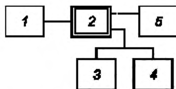
1 — высокочастотный генератор сигналов; 2 — испытываемое оборудование; 3 — вольтметр переменного тока; 4 — эквивалент нагрузки; 5 — анализатор спектра
