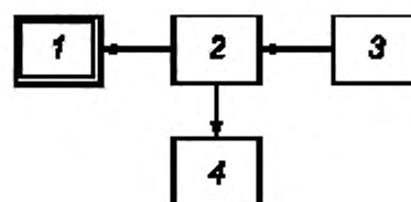
1 — испытываемое оборудование; 2 — делитель мощности; 3 — высокочастотный генератор сигналов; 4 — анализатор спектра
