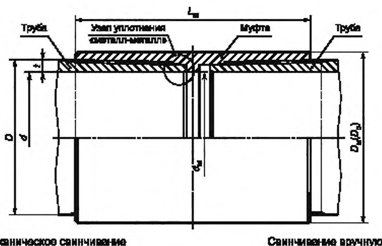
Рисунок 6 — Общий вид резьбового соединения ОТТГ
