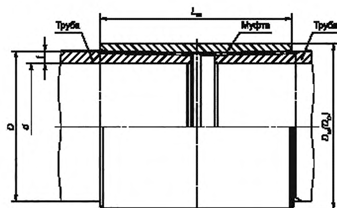
Механическое соединение
