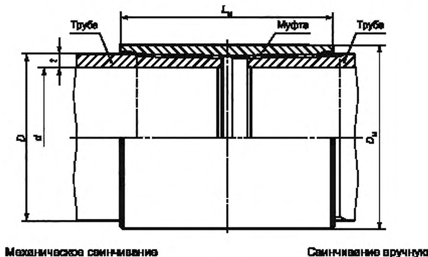
Рисунок 13 — Общий вид резьбового соединения НКТ
