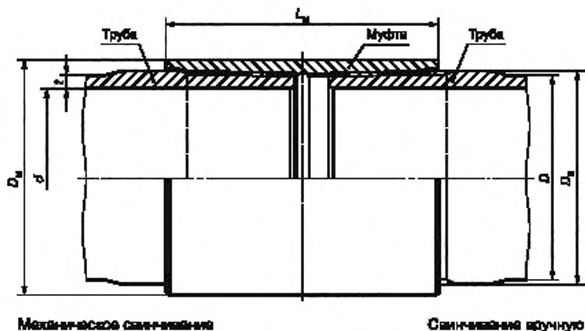
Рисунок 13 — Общий вид резьбового соединения НКТ
