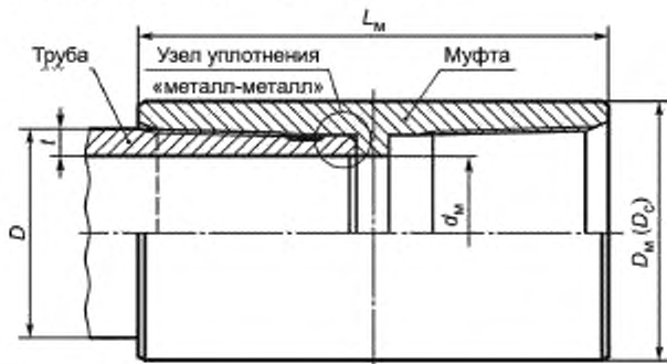
A — натяг при свинчивании труб с муфтами вручную Рисунок 17 — Свинчивание муфты и трубы с резьбовыми соединениями НКТ или НКТВ
