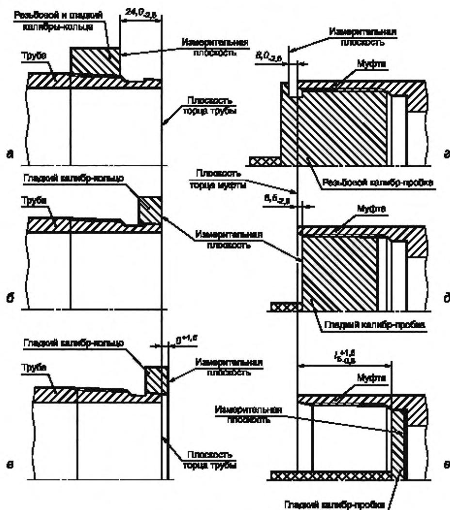
Рисунок 23 — Схема контроля калибрами резьбового соединения ОТГ
