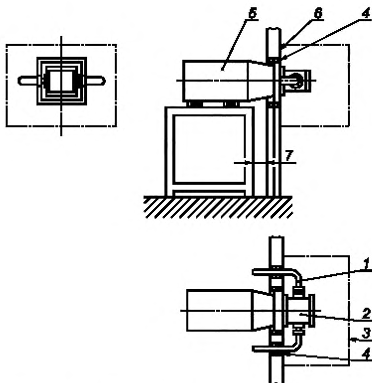
Рисунок 4 — Звукоотражающая плоскость, проходящая через плоскость разреза по монтажному фланцу, при жесткой станине приводного двигателя и трубопроводах, проходящих через звукоотражающую плоскость
