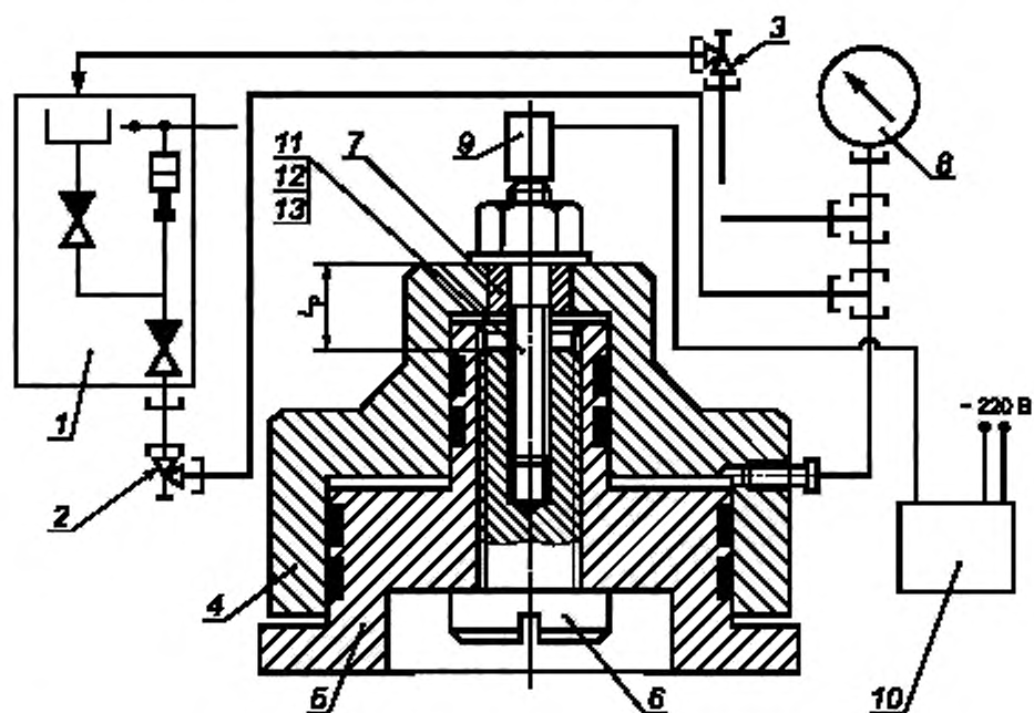
Принципиальная схема гидравлического градуировочного стенда
