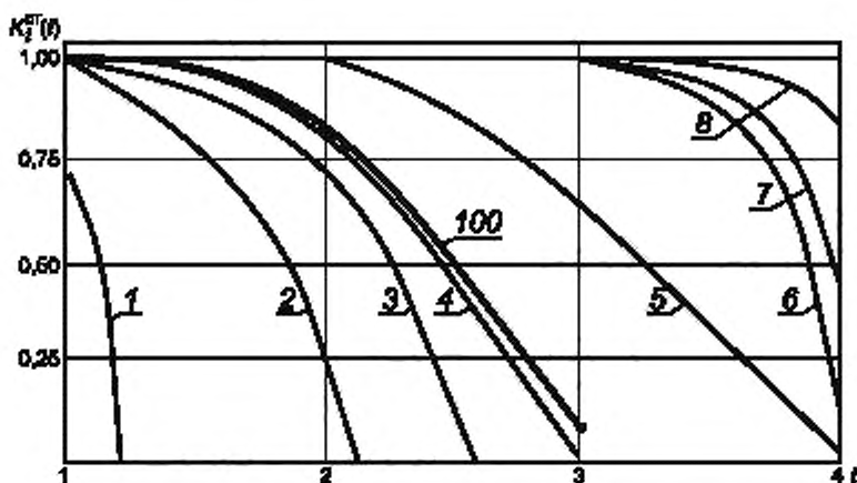
Рисунок А.2 — Кривая зависимости K_f(l) , нанесенная на серию тарировочных кривых
