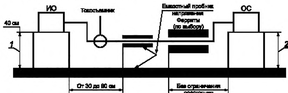
Рисунок А.3 — Испытательная установка
