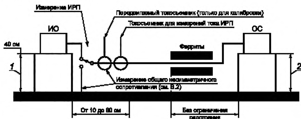
Рисунок А.4 — Испытательная установка
