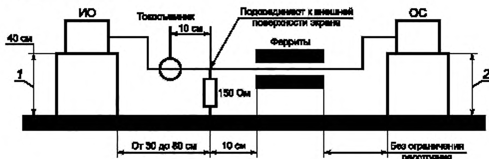
Рисунок А.2 — Испытательная установка ПЭМИН
