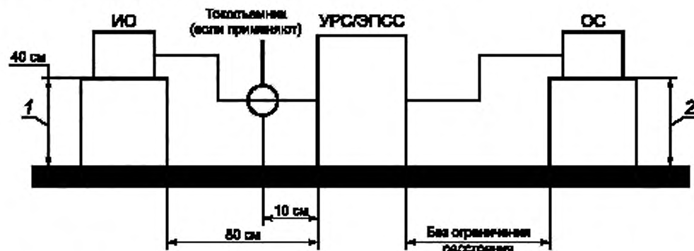
Рисунок А.1 — Испытательная установка ПЭМИН
