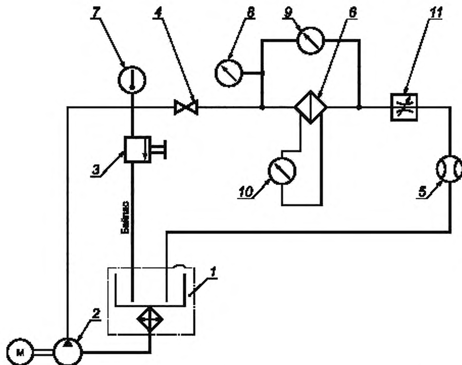
1 — бак (желательно теплоизолированный), имеющий подогреватель и охладитель с собственными термостатами; 2 — насос с приводом; 3 — дроссельный клапан; 4 — отсечной клапан; 5 — расходомер; 6 — испытываемый фильтр; 7 — датчик температуры, соединенный с индикатором температуры; 8 — манометр; 9 — дифференциальный манометр или два обычных манометра для измерения перепада давления на фильтре; 10 — дифференциальный манометр или два обычных манометра для измерения перепада давления на фильтрующем элементе; 11 — дроссельный клапан
