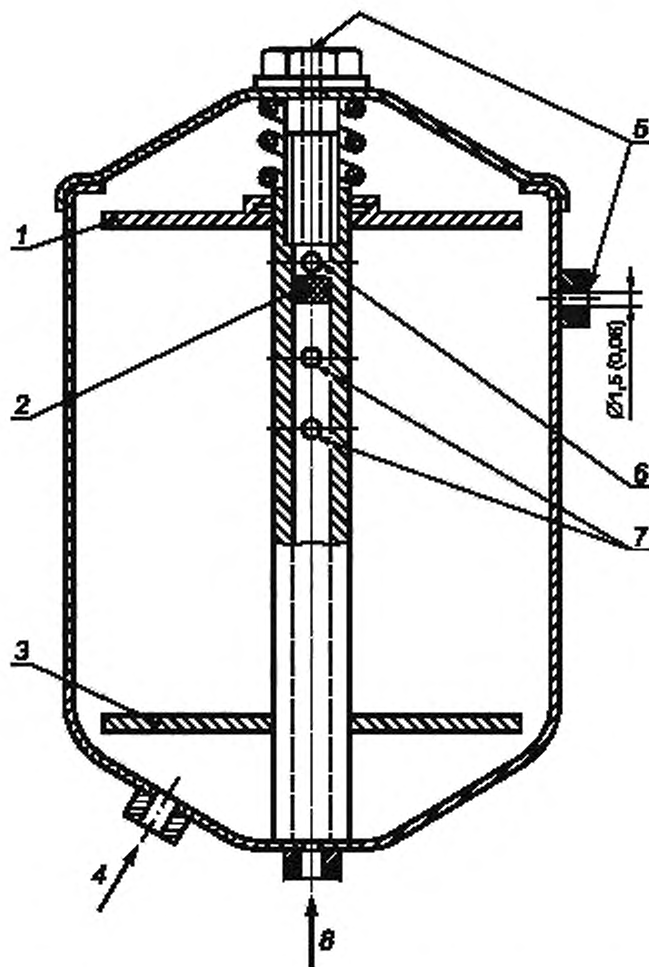
1 — верхняя (подвижная) пластина с уплотнением вокруг центральной трубки; 2 — заглушка в центральной трубке; 3 — опорная (неподвижная) пластина с уплотнением вокруг центральной трубки; 4 — вход; 5 — штуцеры для измерения перепада давления на фильтрующем элементе; 6 — отверстия, защищенные от заусениц; 7 — отверстия в центральной трубке с общим проходным сечением не менее 1,5 площади проходного сечения входного отверстия; 8 — выход
