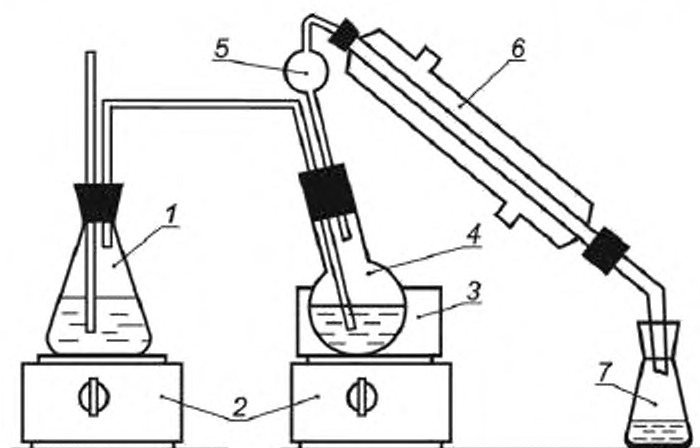
1 — колба коническая вместимостью 500 см 3 ; 2 — плита электрическая; 3 — баня с насыщенным раствором хлористого натрия; 4 — колба для отгонки аммиака с паром; 5 — каплеуловитель; 6 — холодильник; 7 — приемная колба (колба коническая вместимостью 250 см 3 )
