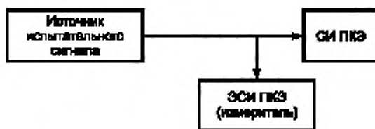
Рисунок 2 — Определение МХ СИ ПКЭ с использованием эталонного измерителя ПКЭ
