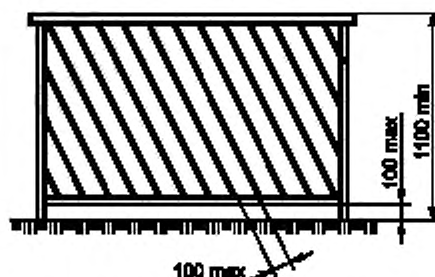
а) Ограждение с вертикальным расположением внутренних элементов
