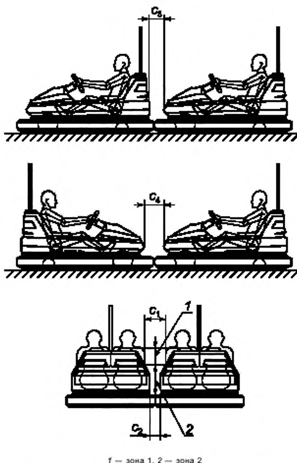
Рисунок 15 — Сталкивающиеся автомобили, лист 1
