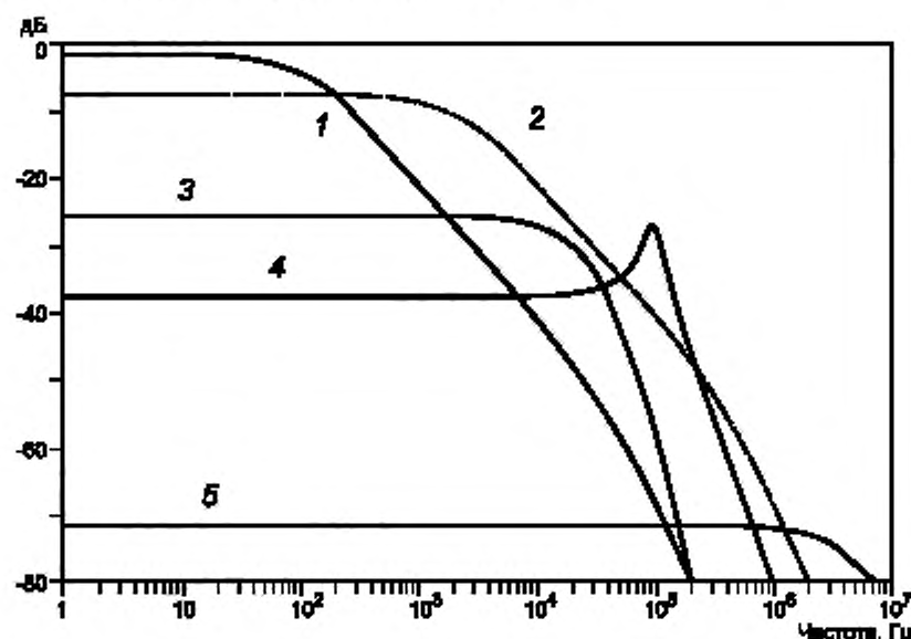
1 — испытательный сигнал 10 мкс (длительность фронта)/1000 мкс (длительность импульса); 2 — микросекундная импульсная помеха большой энергии (импульс напряжения 1/50 мкс) (см. ГОСТ Р 51317.4.5); 3 — микросекундная импульсная помеха большой энергии (импульс тока 6,4/16 мкс) (см. ГОСТ Р 51317.4.5); 4 — одиночная колебательная затухающая помеха с частотой колебаний 100 кГц (см. ГОСТ Р 51317.4.12); 5 — пакеты наносекундных импульсных помех 5/50 нс (см. ГОСТ Р 51317.4.4)
