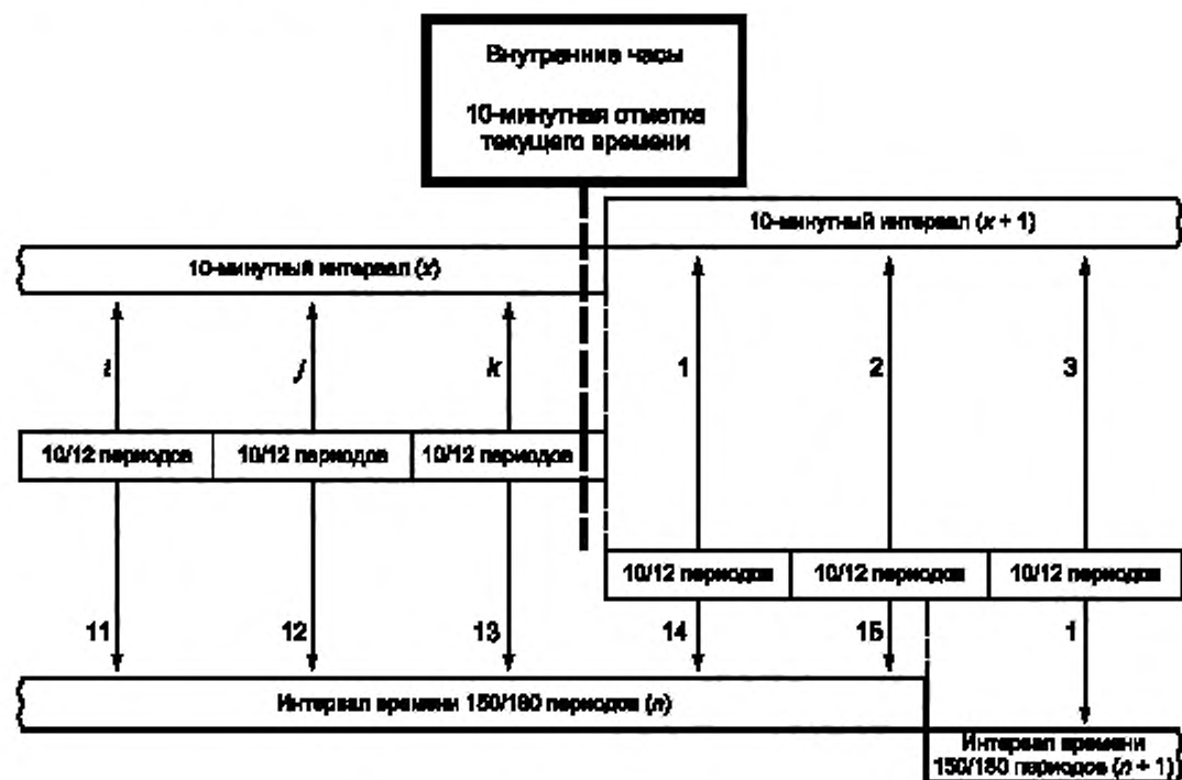
Рисунок 3 — Синхронизация объединенных интервалов для класса S: измерение показателей КЗ, для которых пропуски недопустимы
