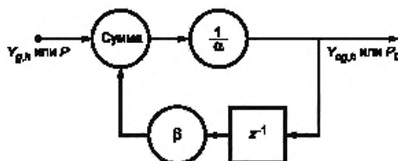
Рисунок 5 — Схема реализации цифрового фильтра низких частот
