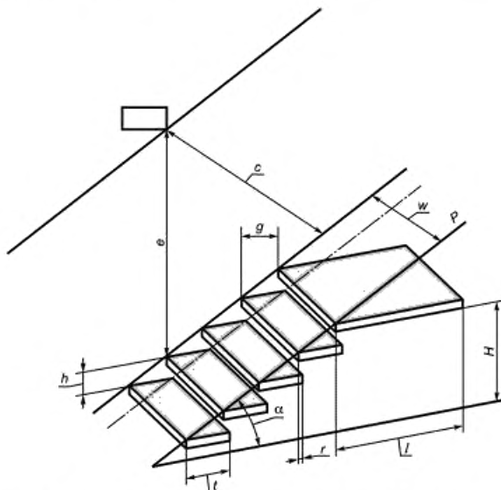
Рисунок 1 — Элементы лестниц
