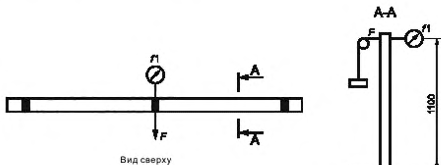
Рисунок 10 — Схема испытания опор
