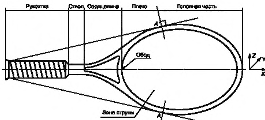
Рисунок 1 — Элементы ракетки
