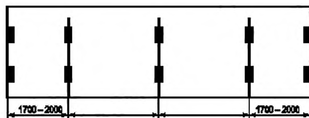
Рисунок В.6 — Контейнеры типов 1EE, 1AA, 1A или 1AX (без тоннеля для установки на полуприцепе с передней балкой типа «шея гуся»). Минимальные требования: пять пар опорных (контактных) площадок (одна пара на каждом торце плюс три промежуточные пары)
