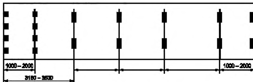
Минимально локализуемая конструкция (см. также рисунок В.10) Рисунок В.9 — Контейнеры типов 1ЕЕЕ, 1ЕЕ, 1ААА, 1АА или 1АХ, имеющие сквозной тоннель для установки на полуприцепе с передней балкой типа «шея гуся». Требования к контейнерам, имеющим семь пар опорных (контактных) площадок
