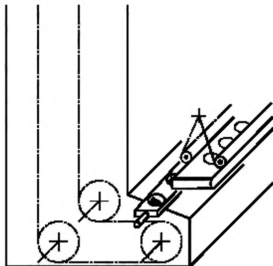
Рисунок 12 — Выталкивающее устройство
