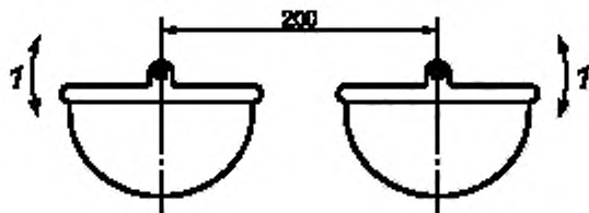
1 — наклоняющиеся люльки
