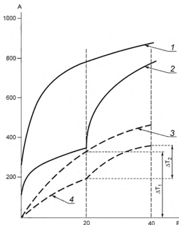
Рисунок Г.1 — Графическое отображение результатов испытаний колонн, проведенных по стандартной кривой и кривой тлеющего пожара
