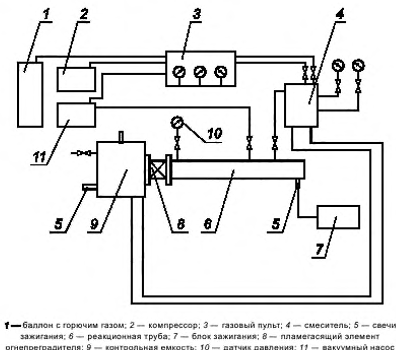
Рисунок 1 — Принципиальная схема экспериментального стенда
