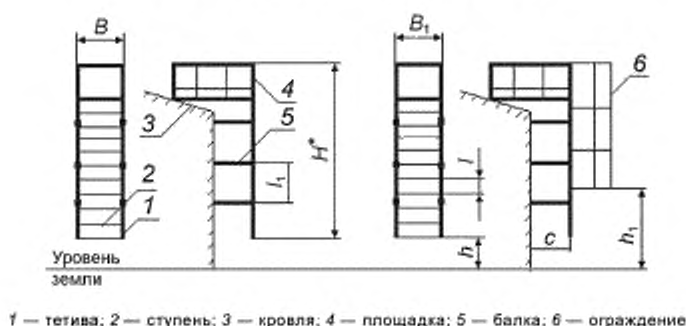
Рисунок Б.1 — Вертикальные лестницы
