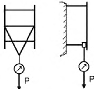
Рисунок Д.2 — Балки
