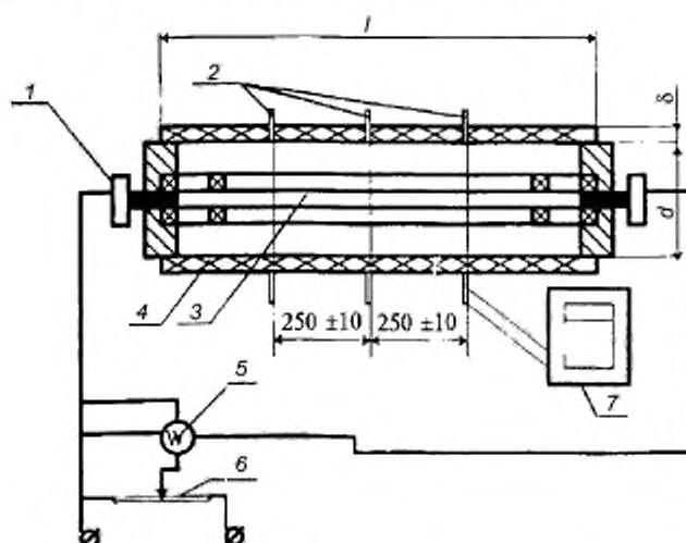
1 — токопроводящая втулка; 2 — термоэлектрические преобразователи; 3 — электронагреватель; 4 — испытываемый материал; 5 — прибор контроля мощности (А, В); 6 — автотрансформатор; 7 — потенциометр
