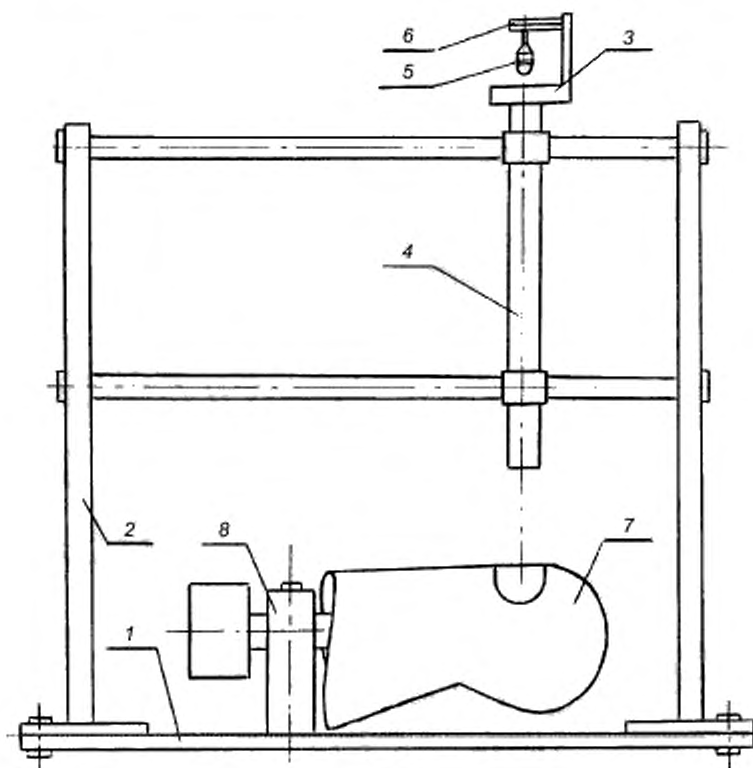
1 — станина; 2 — стойки; 3 — держатель; 4 — направляющая труба; 5 — ударник; 6 — спусковое устройство; 7 — испытуемое средство защиты головы; 8 — устройство для закрепления испытуемого средства защиты
