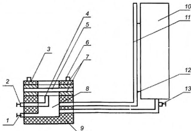
1 — сливной кран; 2 — кран для удаления воздуха из испытательной камеры; 3 — кольцо для зажима образца; 4 — трубка для определения уровня воды в испытательной камере и слива; 5 — образец; 6 — «гайки-барашки»; 7 — резиновые прокладки; 8 — испытательная камера; 9 — основание камеры; 10 — емкость с водой, создающая давление на образец; 11 — трубка со шкалой делений для измерения давления на образец; 12 — крепление трубки со шкалой делений к емкости с водой; 13 — кран подачи воды в испытательную камеру
