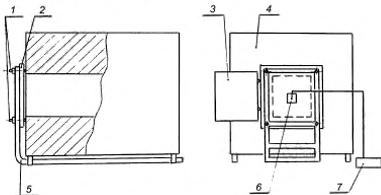
1 — испытуемый образец; 2 — шпильки; 3 — держатель образца; 4 — дверь камеры; 5 — электроды; 6 — термоэлектрический преобразователь; 7 — измеритель температуры
